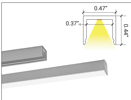
LP-LGC-CM-050/ Surface
