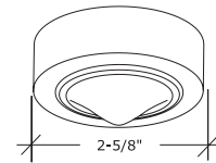
HU-08-3 LED-HU-08-3
