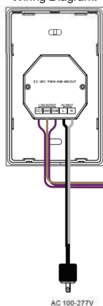
Wiring Diagram:
