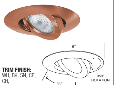
B1663CP PAR36 GIMBAL RING
